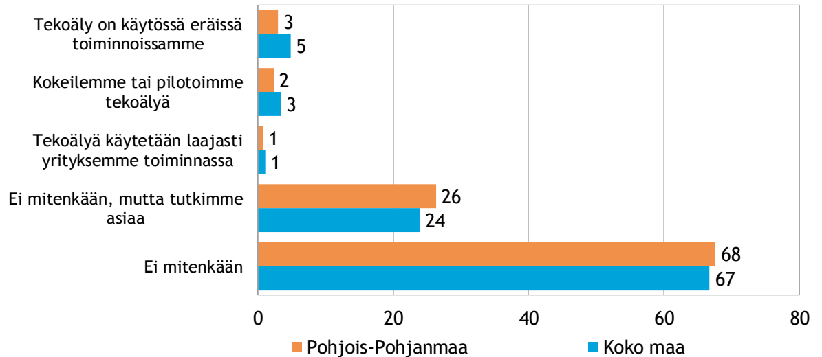
Kuva 22. Tekoälyn hyödyntäminen, %
