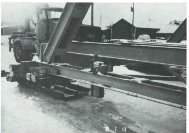
Sillan siirto paikalle tapahtui neljän anturan varassa. Siirtorata oli jäädytetty, jolloin kaivinkoneen ja auton voimat riittivät siirtoon.
