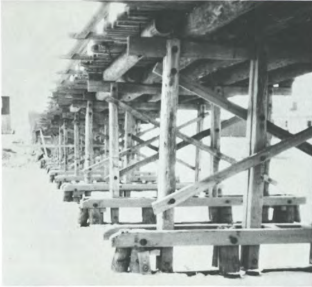
Akkaansilta oli puuta. Viimeinen painorajoitus oli 4 tonnia ja nopeusrajoitus 10 km tunnissa.
